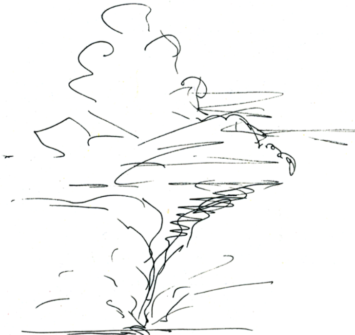
Wirbelsturm
